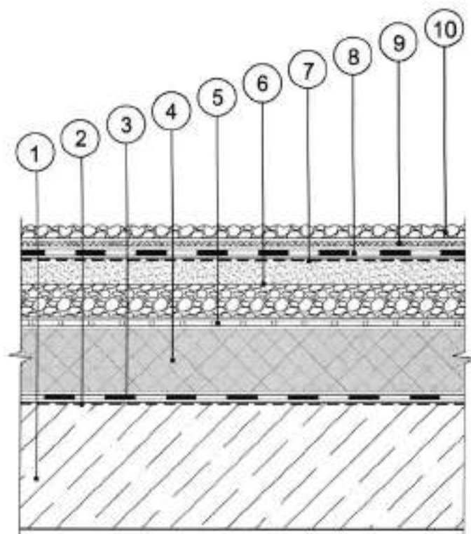
Рис. 4. Кровельная система № 4
