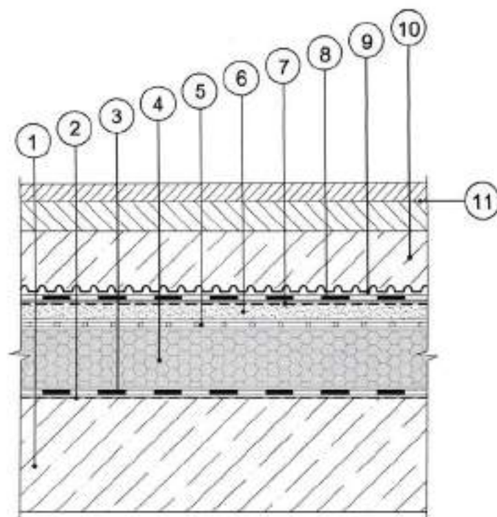
Рис. 9. Кровельная система № 9
