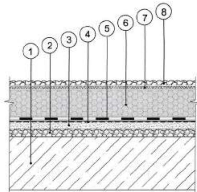
Рис. 11. Кровельная система № 11
