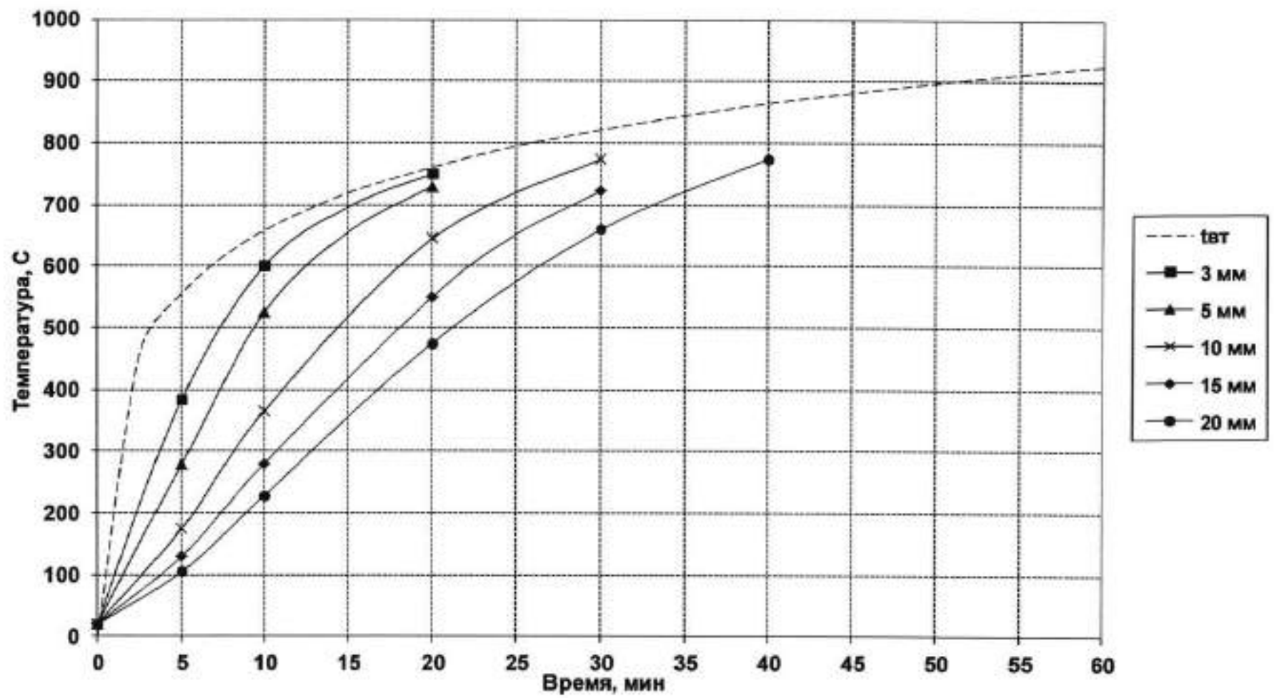
Рис. 19. Номограмма прогрева незащищенных стальных конструкций
