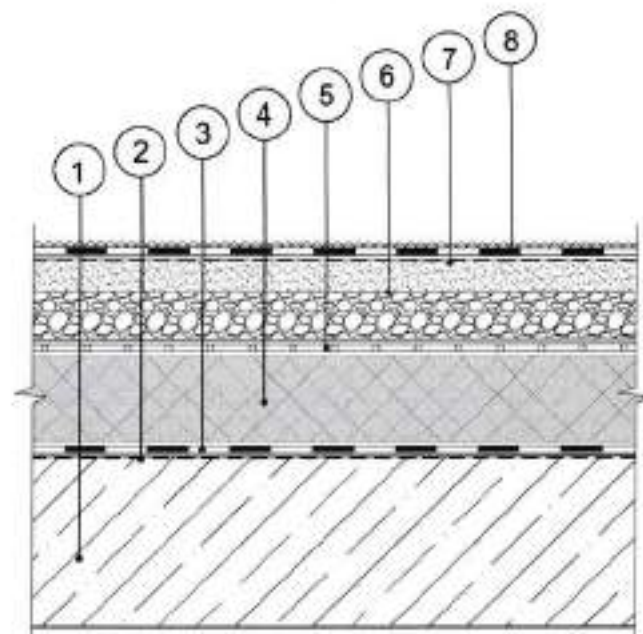
Рис. 1 Кровельная система № 1
