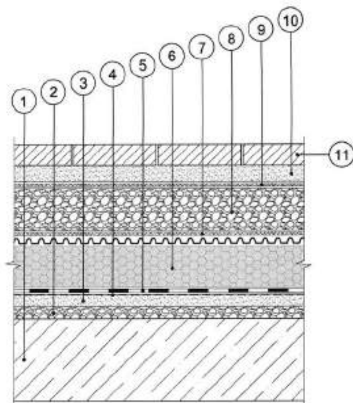
Рис. 12. Кровельная система № 12
