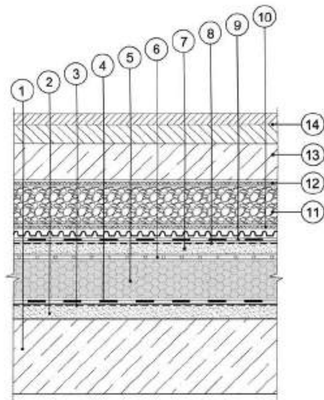
Рис. 8. Кровельная система № 8
