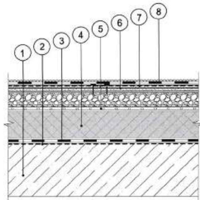
Рис. 2. Кровельная система № 2
