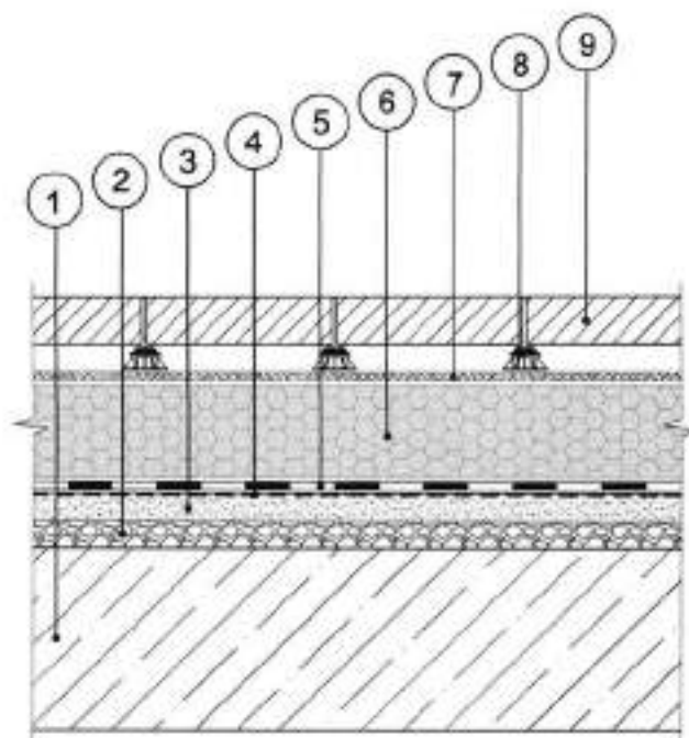
Рис. 10. Кровельная система № 10
