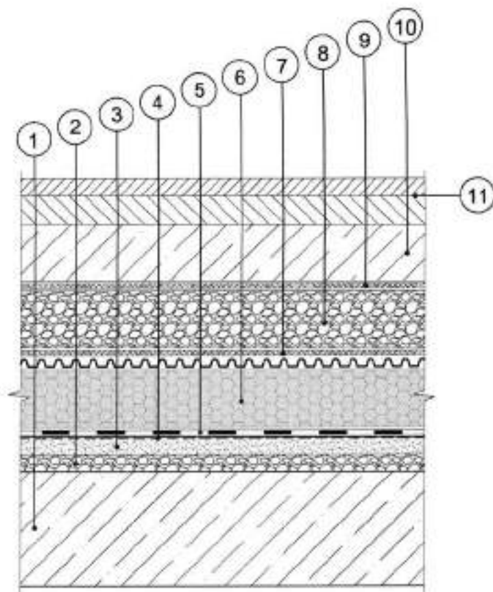
Рис. 13. Кровельная система № 13
