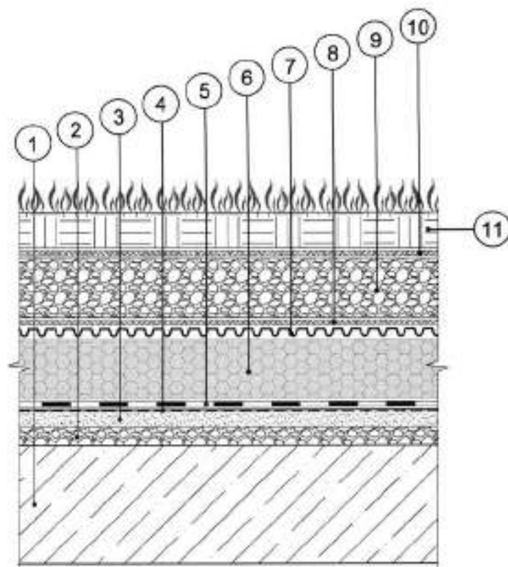
Рис. 14. Кровельная система № 14
