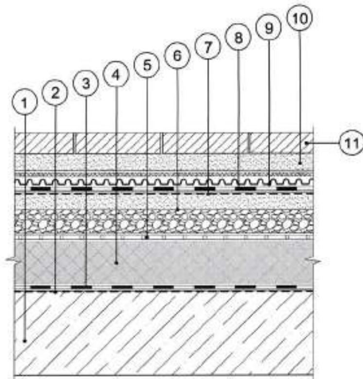
Рис. 6. Кровельная система № 6
