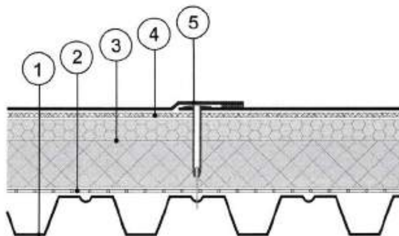
Рис. 17. Кровельная система №17
